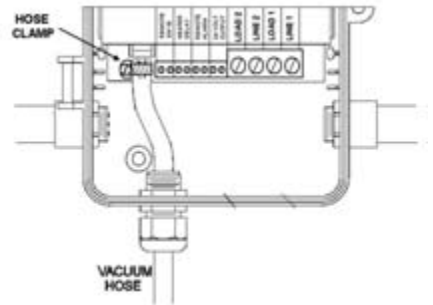
Fig. 2.A: Hose Clamp
